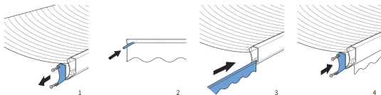
fig. 6.1 Plaatsen volant
