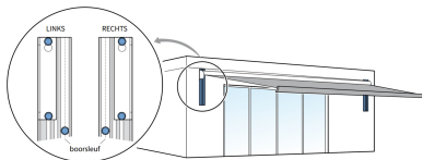
fig. 1.3 Toepassing van muurstrips
