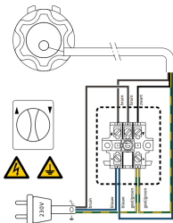
fig. 2.1 Motor links (van buitenaf gezien)
