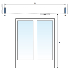
fig. 1.2 Plaatsing muursteunen
