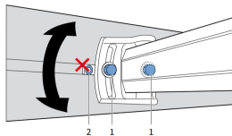
fig. 5.2 Detail armverbinding op voorlijst
