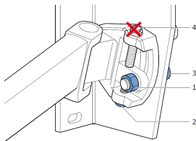
fig. 4.1 Detail armverbinding rechts
