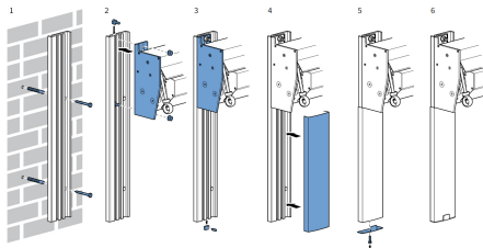
fig. 1.4 Montage van muurstrip (links)
