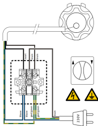
fig. 2.2 Motor rechts (van buitenaf gezien)
